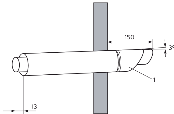
Detail vodorovného odkouření
